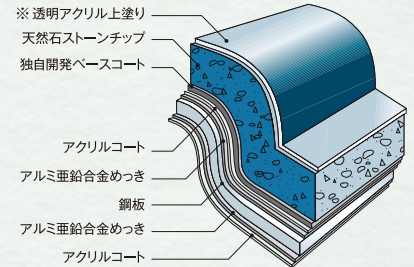
断面構成図
